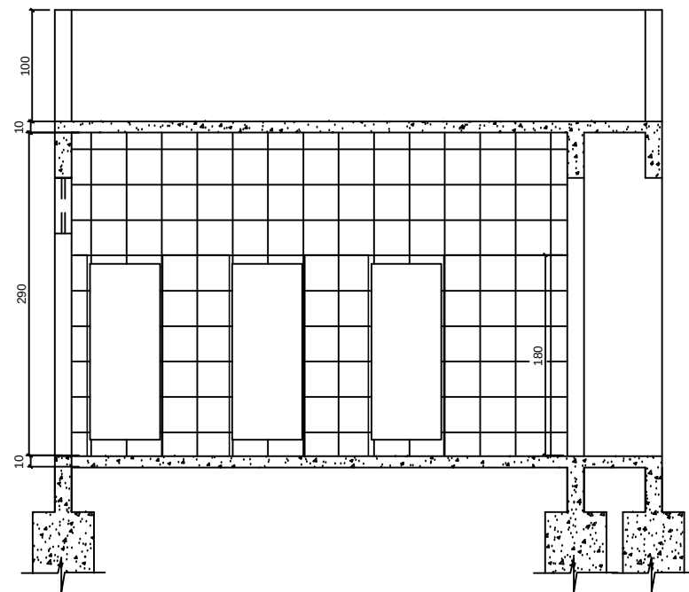
CORTE B-B
