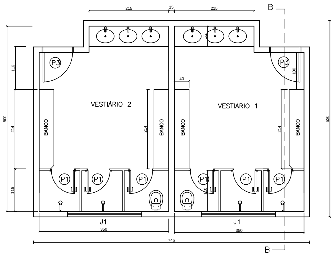
PLANTA BAIXA
